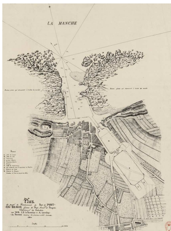
Plan du projet de rétablissement du port de Port-en-Bessin,... / par MM. L.E. Le Forestier et A. Lavalley-du Perroux, membres de plusieurs sociétés savantes, plan de 1840, gallica.bnf.fr / Bibliothèque nationale de France.
